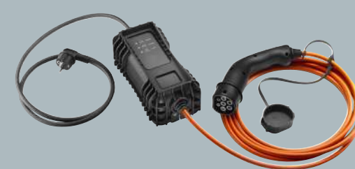
Kabel MODE 2 Dodatna oprema
